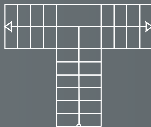
DREILÄUFIG, ZWEIMAL ABGEWINDELT MIT 1 PODEST
