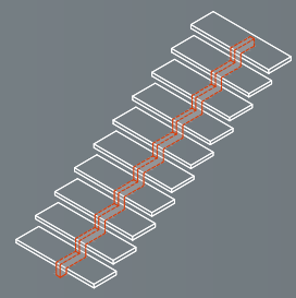
ZENTRALER TRÄGER
