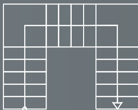
DREILÄUFIG, ZWEIMAL ABGEWINDELT MIT 2 PODESTE
