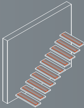
KRAGARMSTUFERN (in der Wand verankert)
